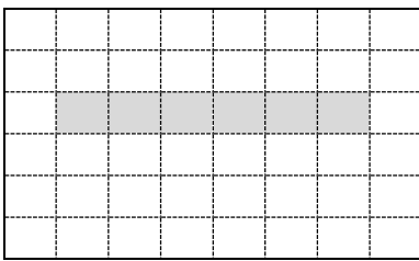
P(3, 2:7) P(3:3, 2:7)
